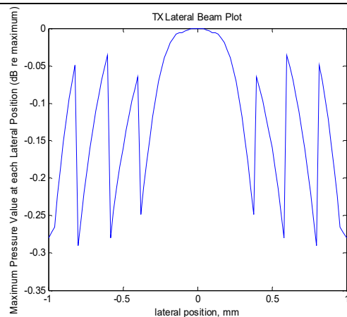
Fig. (d1) TX Lateral beam-plot
